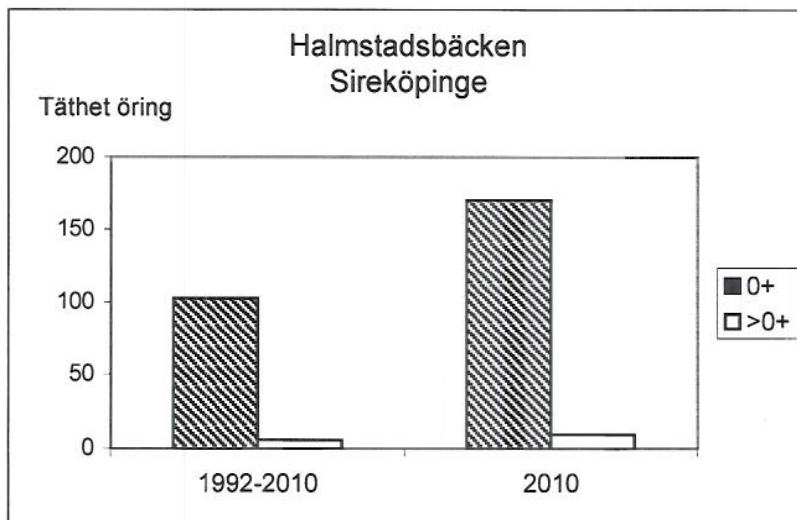
Figur 7. Täthet öring (antal/100 m 2 ), staplar till vänster medelvärde för perioden 1992-2010.
