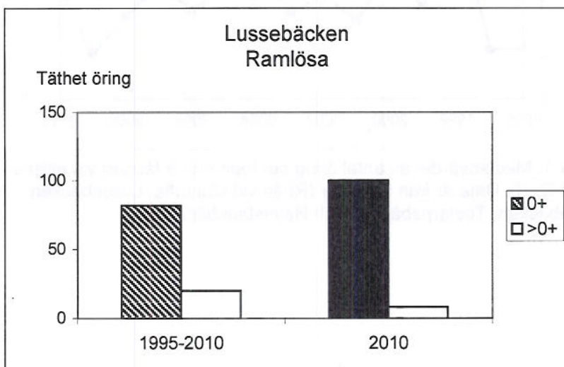
Figur 4. Täthet öring (antal/100 m 2 ), staplar till vänster medelvärde för perioden 1995-2010.
