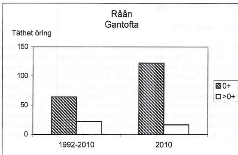
Figur 2. Täthet öring (antal/100 m 2 ), staplar till vänster medelvärde för perioden 1992-2010.
