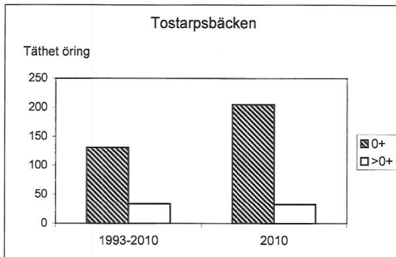
Figur 6. Täthet öring (antal/100 m 2 ), staplar till vänster medelvärde för perioden 1993-2010.
