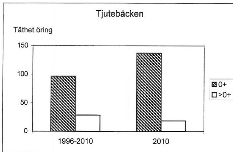
Figur 5. Täthet öring (antal/100 m 2 ), staplar till vänster medelvärde för perioden 1996-2010.
