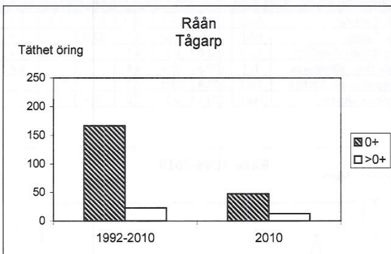
Figur 3. Täthet öring (antal/100 m 2 ), staplar till vänster medelvärde för perioden 1992-2010.
