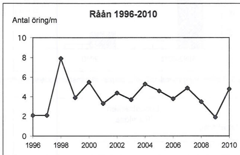
Figur 1. Medianvärdet av antal öring per löpmeter å fångad vid elfiske i Råån 1996-2010. Data är från 5 lokaler (Råån vid Gantofta, Lussebäcken, Tjutebäcken, Tostarpsbäcken och Halmstadsbäcken).
