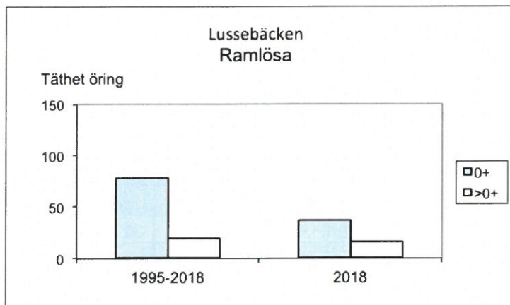
Figur 3. Täthet öring (antal/100 m 2 ), staplar till vänster medelvärde för perioden 1995-2018.
