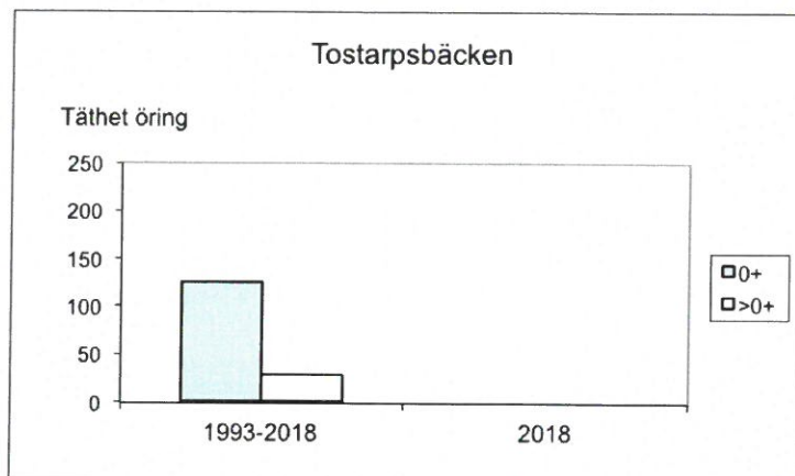
Figur 5. Täthet öring (antal/100 m 2 ), staplar till vänster medelvärde för perioden 1993-2018.
